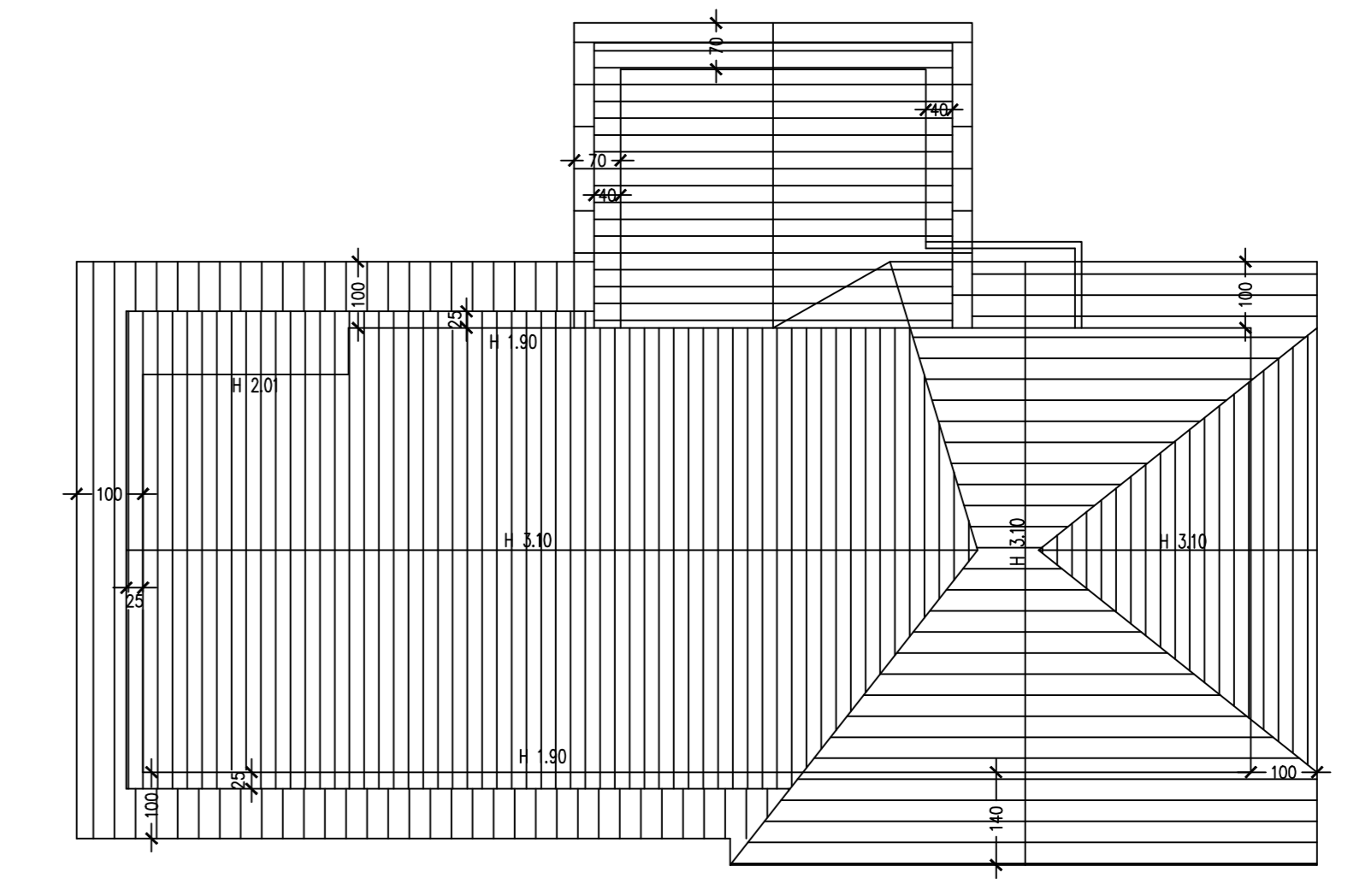
PIANTA COPERTURA
